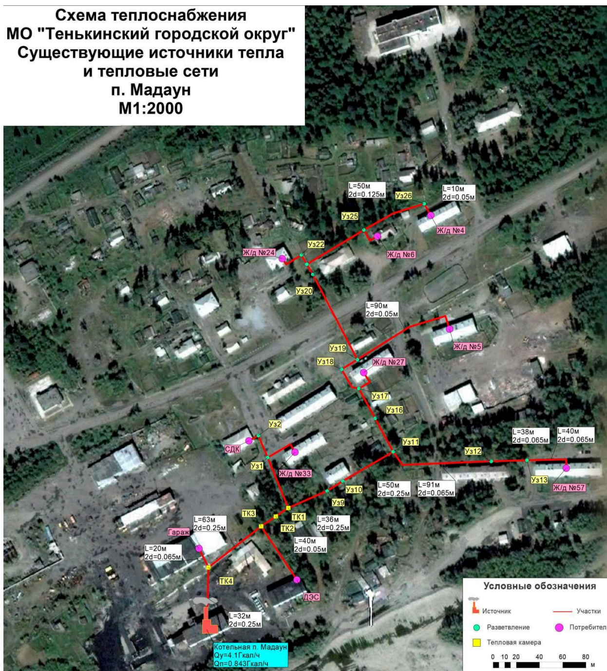
Рисунок 1.3.1 – Схема тепловых сетей п. Мадаун
