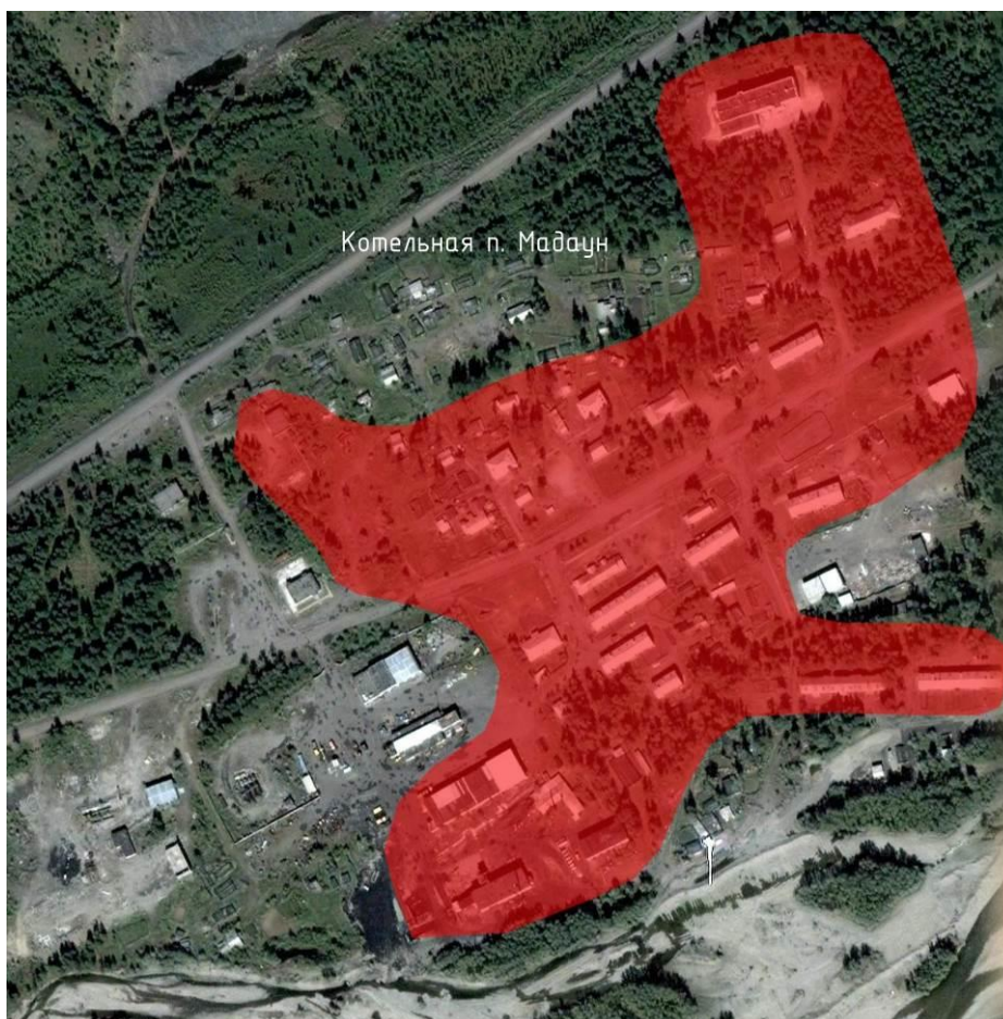
Рисунок 1.1 – Зоны действия систем теплоснабжения п. Мадаун
